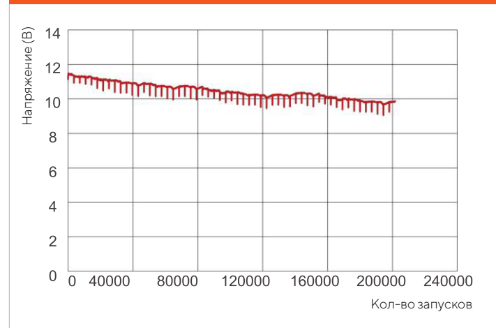
ГРАФИК ИЗНОСА АКБ (25°С)
