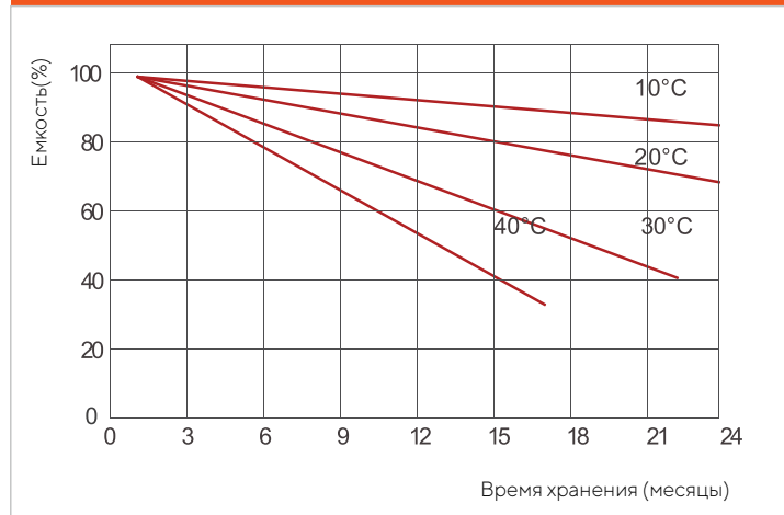
ГРАФИК САМОРАЗРЯДА В ЗАВИСИМОСТИ ОТ ТЕМПЕРАТУРЫ
